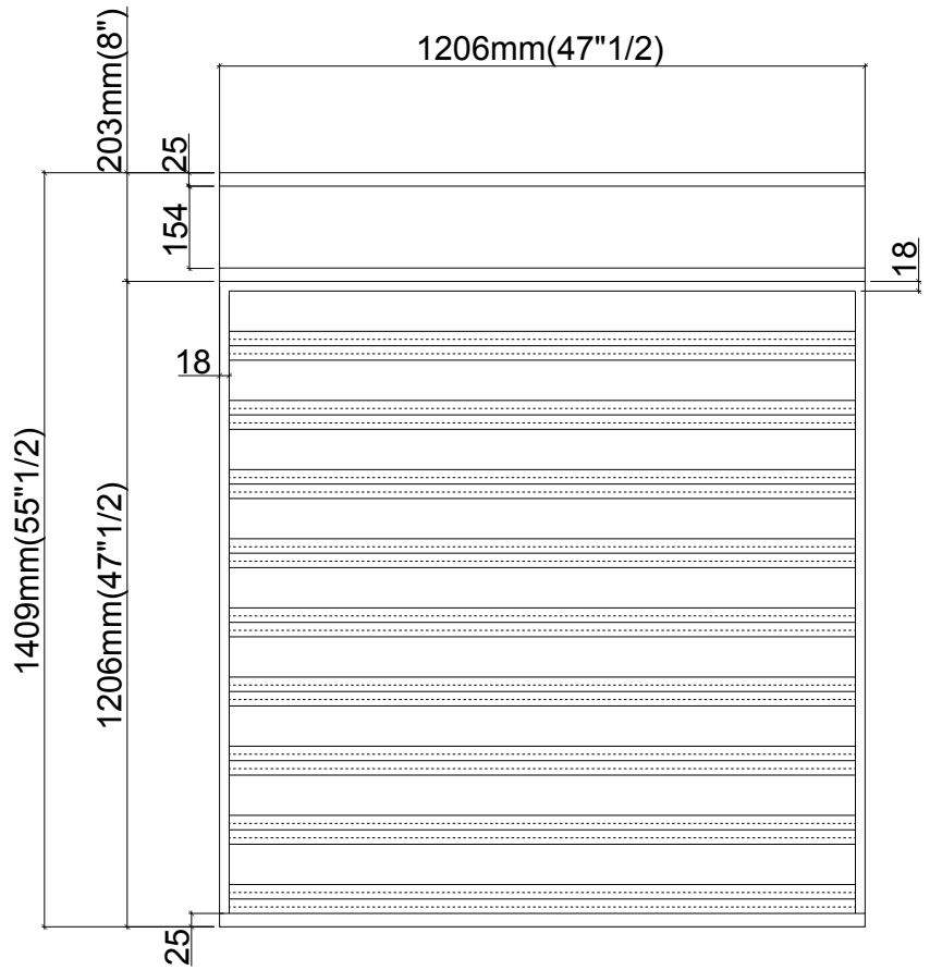
MẶT ĐỨNG
